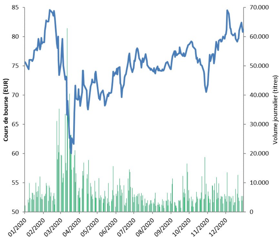
Evolution du cours de bourse de l'action Brederode (EUR) et du volume journalier (nombre de titres) depuis le 1 er janvier 2020
